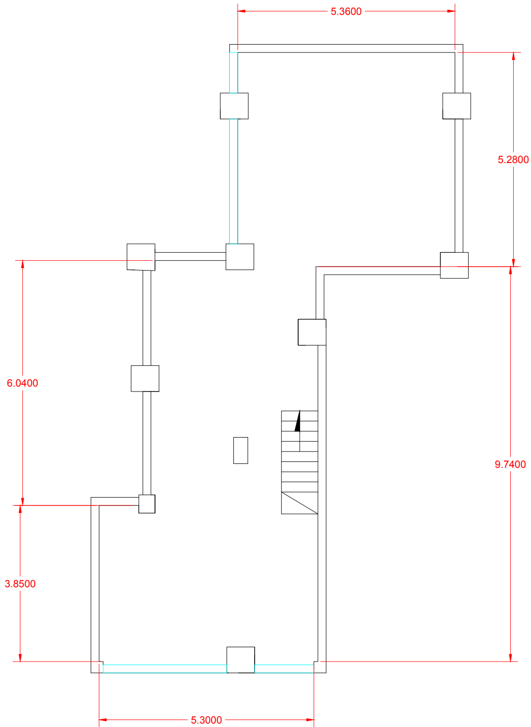
PLANTA ORIGINAL NIVEL ACCESO M2 = 71.35
