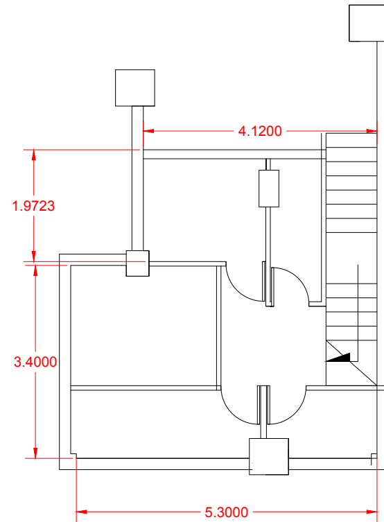
PLANTA ORIGINAL NIVEL ACCESO M2 = 71.35
